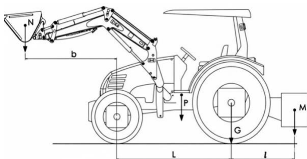
Рисунок 5. Статическая устойчивость системы трактор – погрузчик
