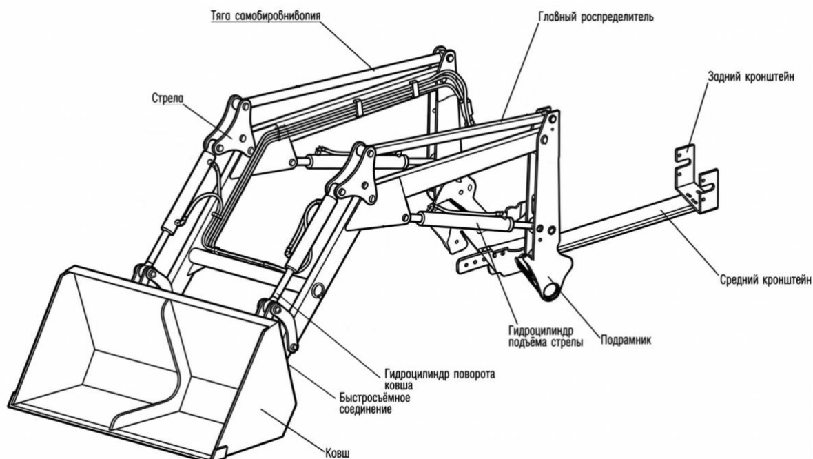
Рисунок 4. Основные элементы конструкции
