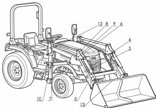
Рисунок 2. Расположение пиктограмм на машине — правая сторона.
